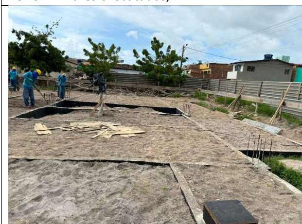
FOTO 3: Aterro executado;
