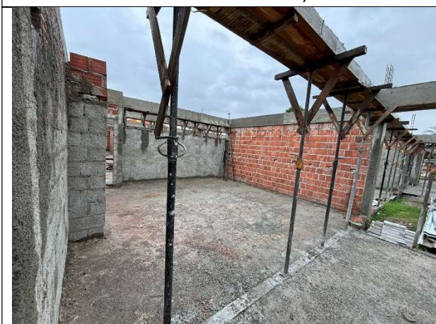
FOTO 5: Alvenaria 1 vez executada;
