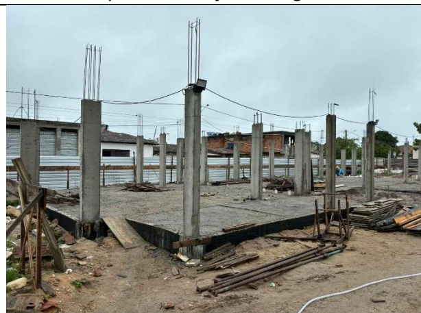
FOTO 16: Lastro de concreto executado;
