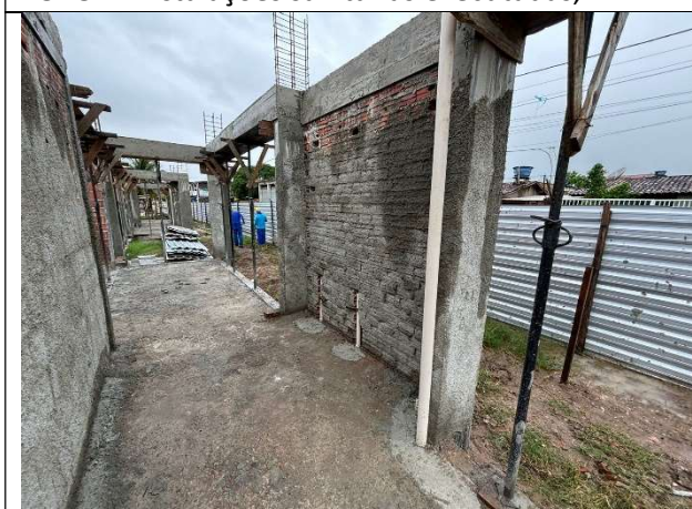
FOTO 9: Instalações sanitárias executadas;
