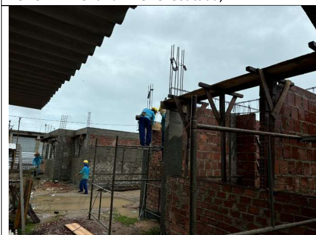
FOTO 3: Alvenaria 1 vez executada;
