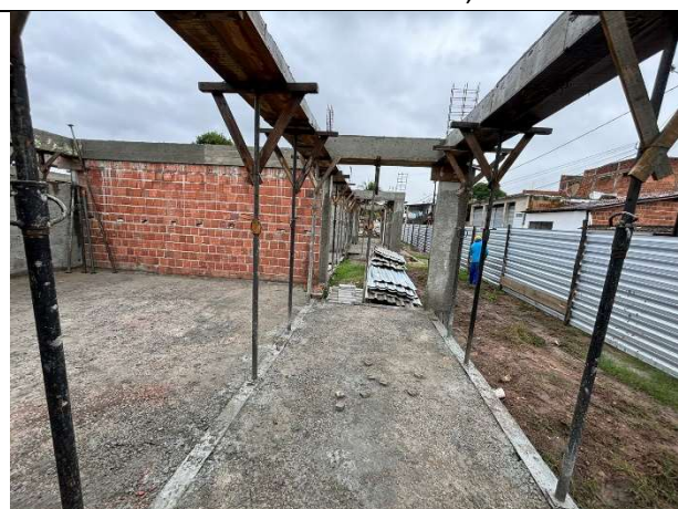
FOTO 6: Alvenaria 1 vez executada;
