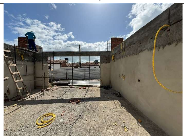
FOTO 10: Eletrodutos instalados;
